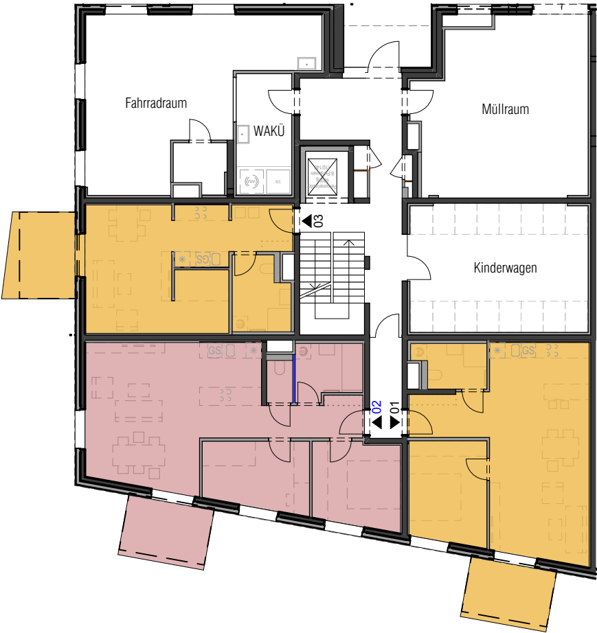
Erdgeschoß
